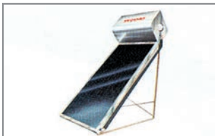
1985 Horizontal storage tank with closed circuit system (with "sandwich" type solar collectors- 120 lt) • Οριζόντια δεξαμενή κλειστού κυκλώματος (με συλλέκτες τύπου "σάντουιτς") (χωρητικότητα 120 lt.)
