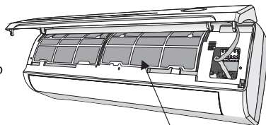
Φίλτρο κατά της σκόνης
