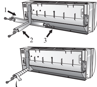
Διαμόρφωση σωλήνα σύνδεσης
