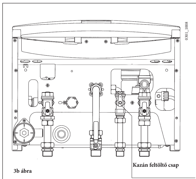
HT 1.120 - HT 1.240 - HT 1.280
