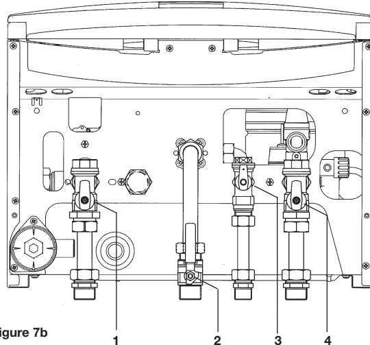
HT 1.120 - HT 1.240 - HT 1.280
