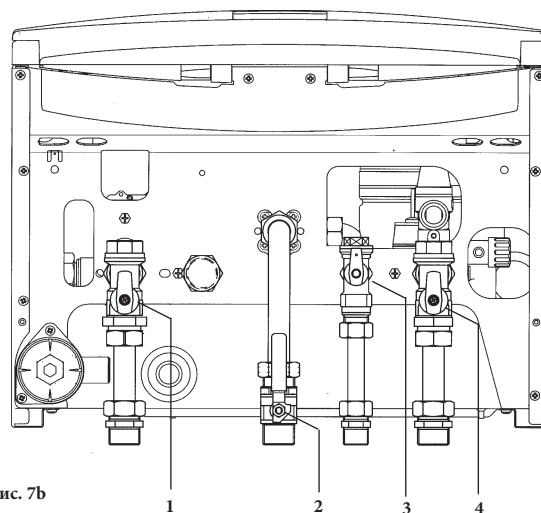
НТ 1.120 - НТ 1.240 - НТ 1.280
